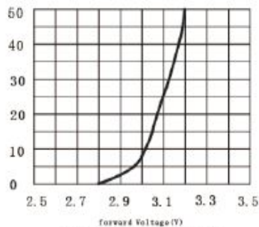
FORWARD CURRENT VS FORWARD VOLTAGE 正向电流和正向电压的关系曲线图
