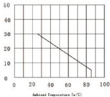
FORWARD CURRENT VS DERATING CURVE 正向电流随温度的曲线图
