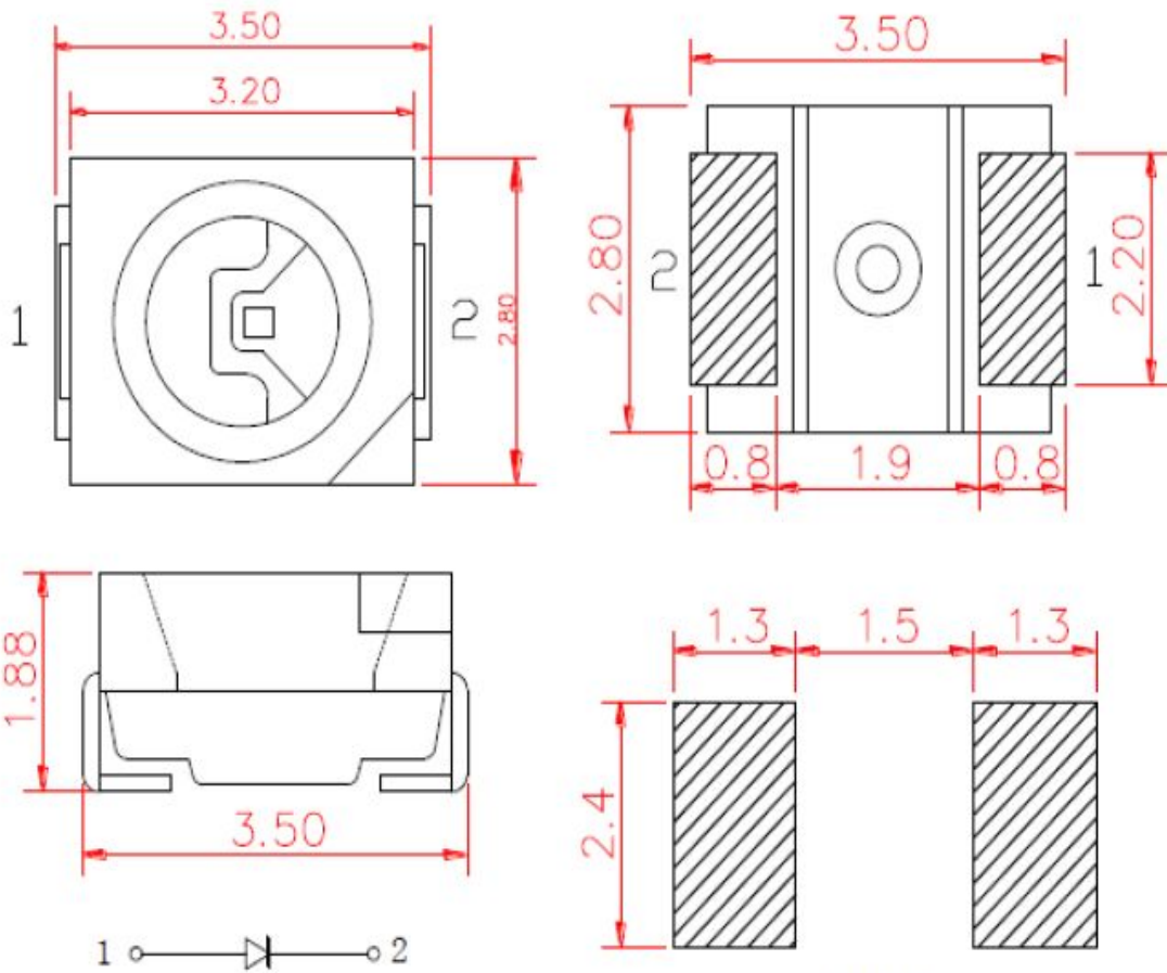
焊盘图
