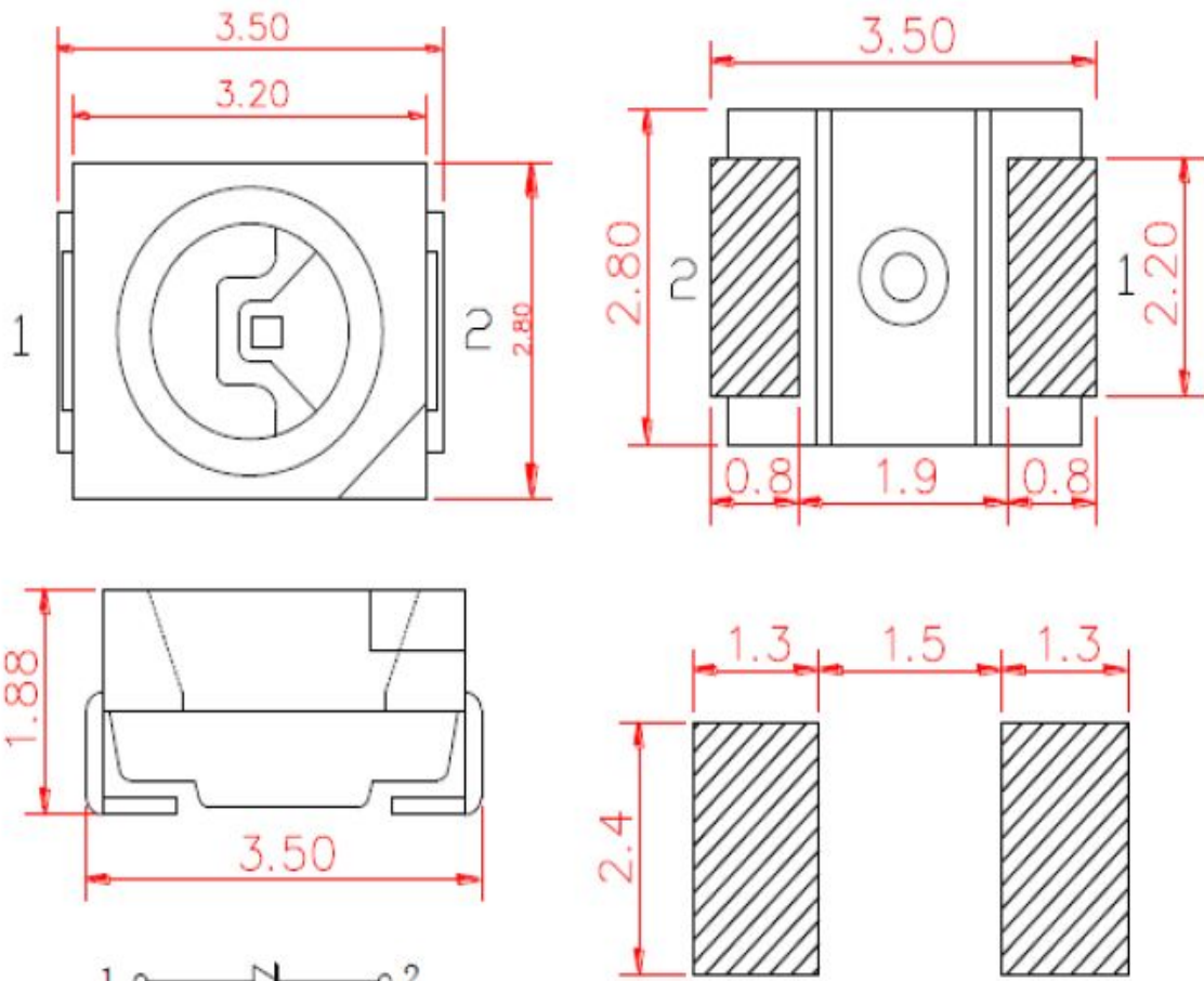
焊盘图
