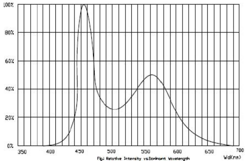
Fig. Relative Intensity vs. Dominant Wavelength 相对亮度与波长之间的关系
