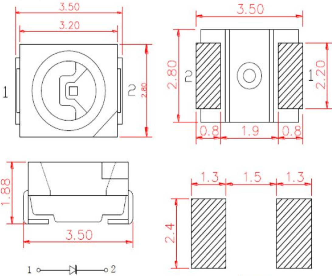
焊盘图
