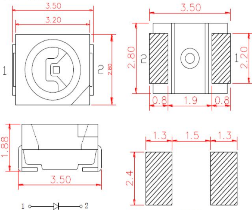
焊盘图
