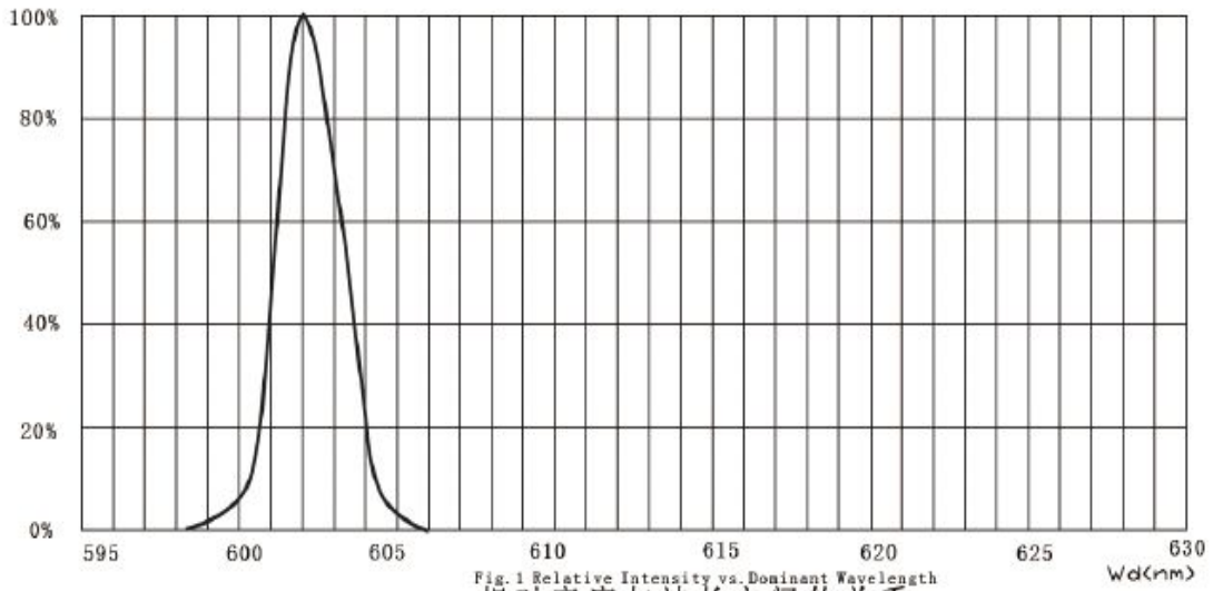
Fig. 1 Relative Intensity vs. Dominant Wavelength 相对亮度与波长之间的关系
